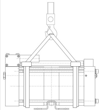
Табл. 5-1 Точки подъема пневматического компрессора
