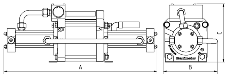
DLE 30 doppeltwirkend, einfacher Luftantrieb, einstufig
