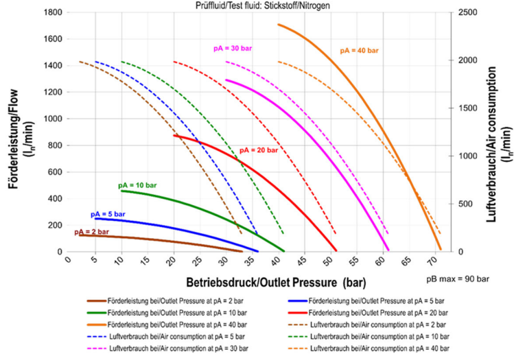
Leistungsdiagramm/Performance Graph GLGP 5 Antriebsdruck/Drive pressure 6 bar Prüffluid/Test fluid: Stickstoff/Nitrogen
