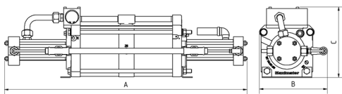
DLE 15-30-2 einfachwirkend, doppelter Luftantrieb, zweistufig
