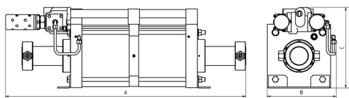
GPD 60-2 doppeltwirkend, doppelter Luftantrieb
