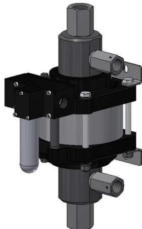
G10D doppeltwirkend, einfacher Luftantrieb (Einlass unten)
