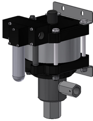
G15 (L) einfachwirkend, einfacher Luftantrieb (Standard=Einlass unten)
