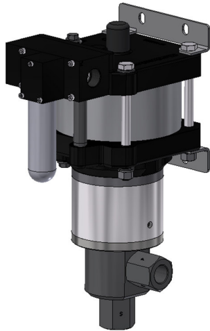
GSF25(L) einfachwirkend, einfacher Luftantrieb mit Distanzstück (Einlass unten)
