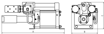
GX35 doppeltwirkend, einfacher Luftantrieb (Einlass unten)
