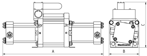
DLE 2 doppeltwirkend, einfacher Luftantrieb, einstufig
