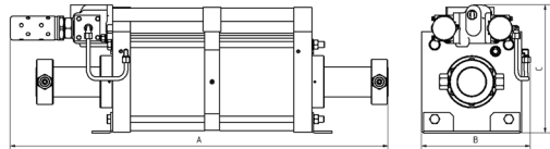
GPD 30-2 doppeltwirkend, doppelter Luftantrieb
