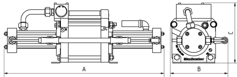
DLE 15-30 einfachwirkend, einfacher Luftantrieb, zweistufig
