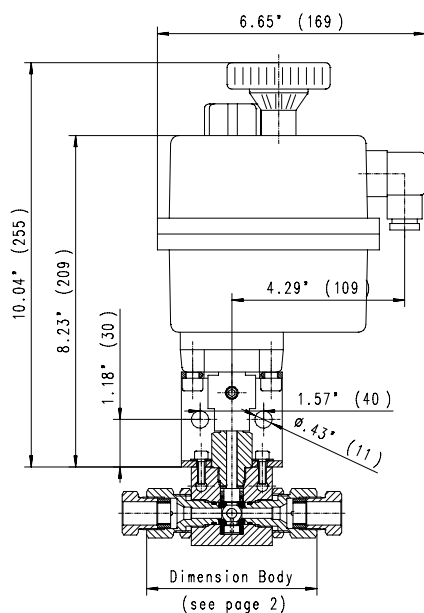
Elektrisch angetriebenes 2-Wege Kugelventil
