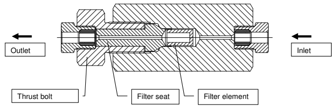
Abb. 14: Prinzip eines Hutfilters
