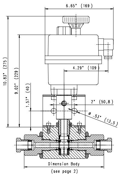
Elektrisch angetriebener 2-Wege-Kugelventil
