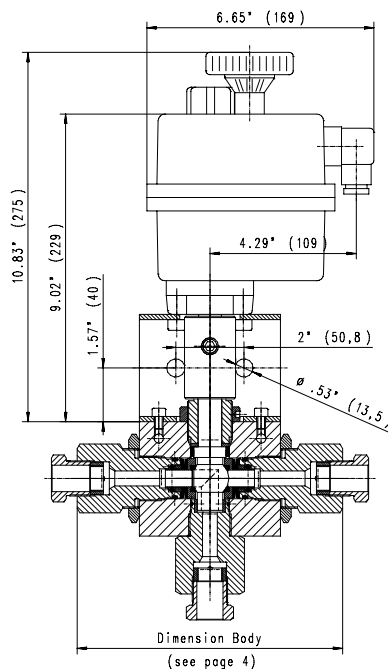
Elektrisch angetriebener 3-Wege-Kugelventil
