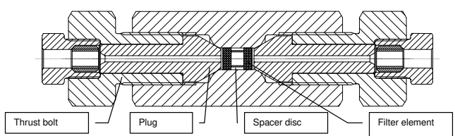
Abb. 13: Prinzip eines Scheibenfilters
