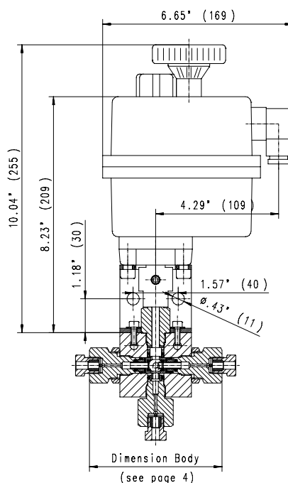
Elektrisch angetriebene 3-Wege-Kugelventil
