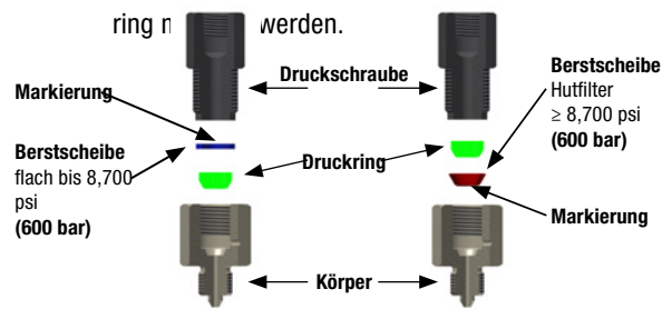
Abb. 12: Berstscheibenformen
