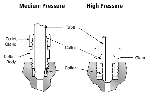
Prinzip einer Antivibrationsverschraubung
