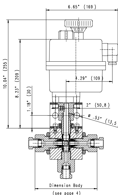
Elektrisch angetriebener 3-Wege-Kugelventil
