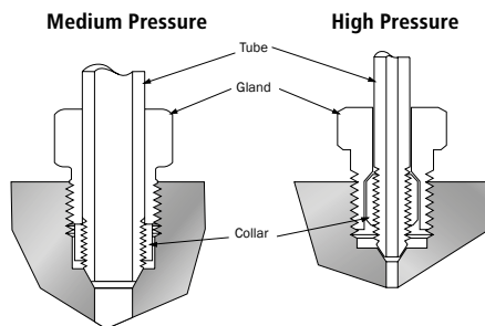
Prinzip einer Hochdruck Verschraubung
