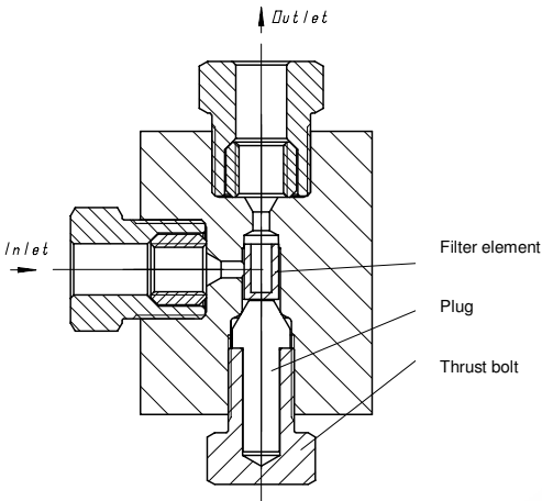
Figure 15: Prinzip eines Winkelfilters
