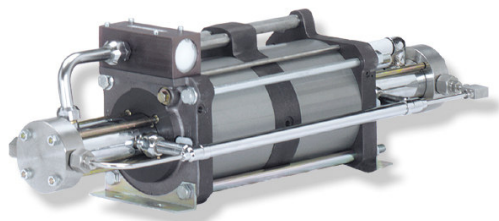
DLE 30-75-2 einfachwirkend, doppelter Luftantrieb, zweistufig
