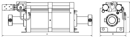
GPD 180-2 doppeltwirkend, doppelter Luftantrieb
