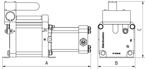
DLE 2-1 einfachwirkend, einfacher Luftantrieb, einstufig
